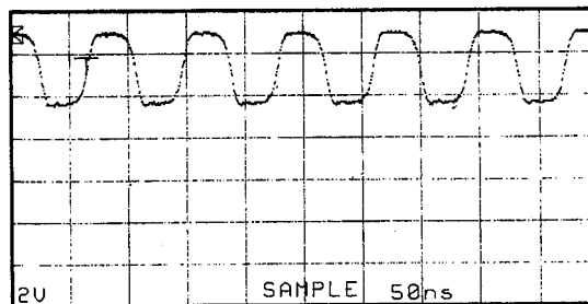
Point ⑥ (Pin 82 of IC 13)
