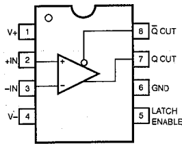
IC2 : LT1016IN8
